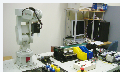
▲ロボット制御実験装置
