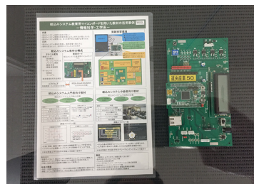
▲組み込みシステム教育用マイコンボード TECL
