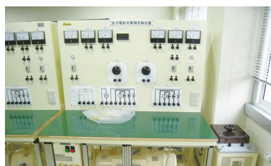
▲直流電動発電機実験設備
