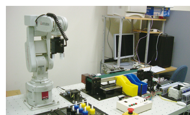
▲ロボット制御実験装置
