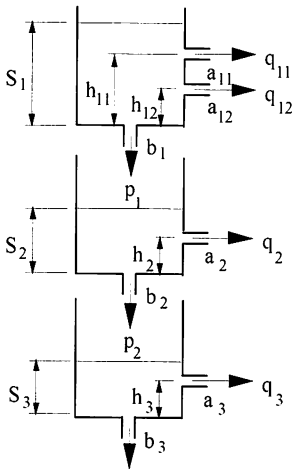
図-5 採用したタンクモデル
