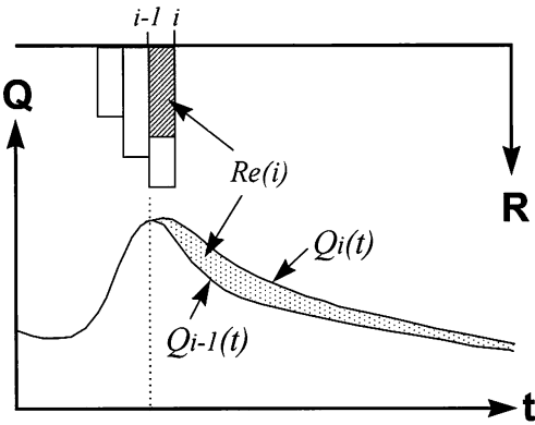
図-7 流出モデルを用いた有効雨量の分離方法
