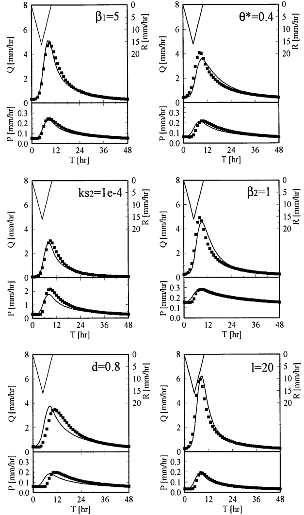
図-13 損失を考慮した貯留型流出モデルによる流出量と損失量の計算結果 (初期条件は全層湿潤後 48 時間の自然排水; 図中の実線は損失を考慮した貯留関数, ■ は不飽和浸透理論による結果)
