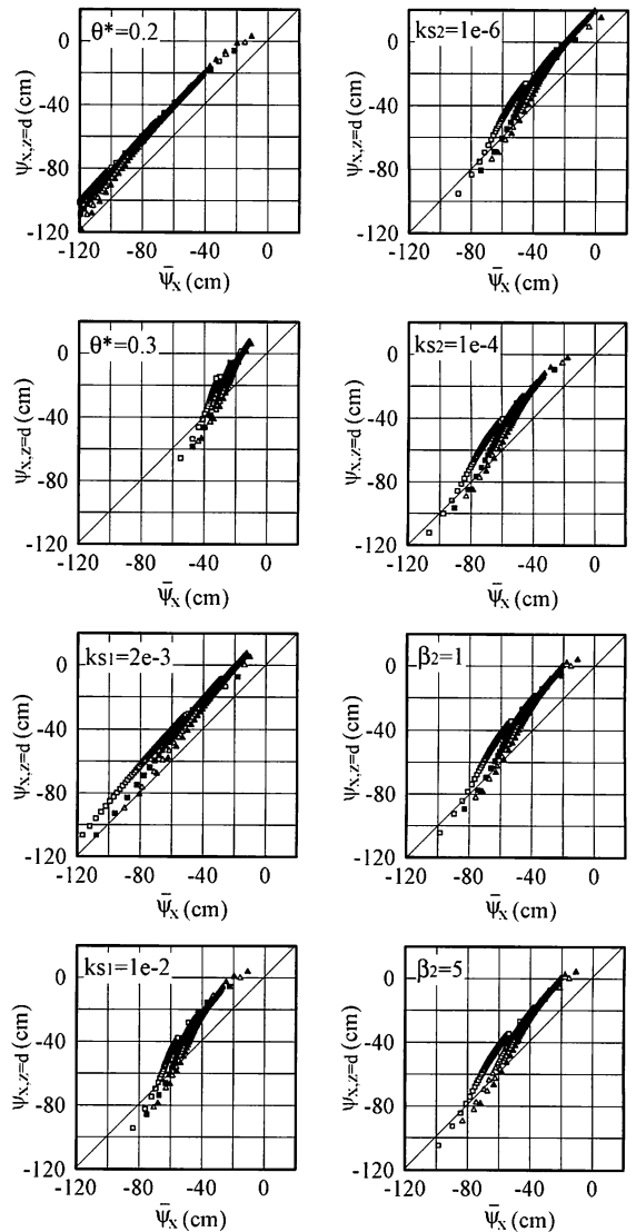
図-11 圧力水頭の断面平均値と浸透層底部の圧力水頭の関係の例(図中の記号□, ■, △, ▲はそれぞれ、0.5, 2.0, 4.0, 6.0mm/hrの定常降雨による計算結果を示す)
