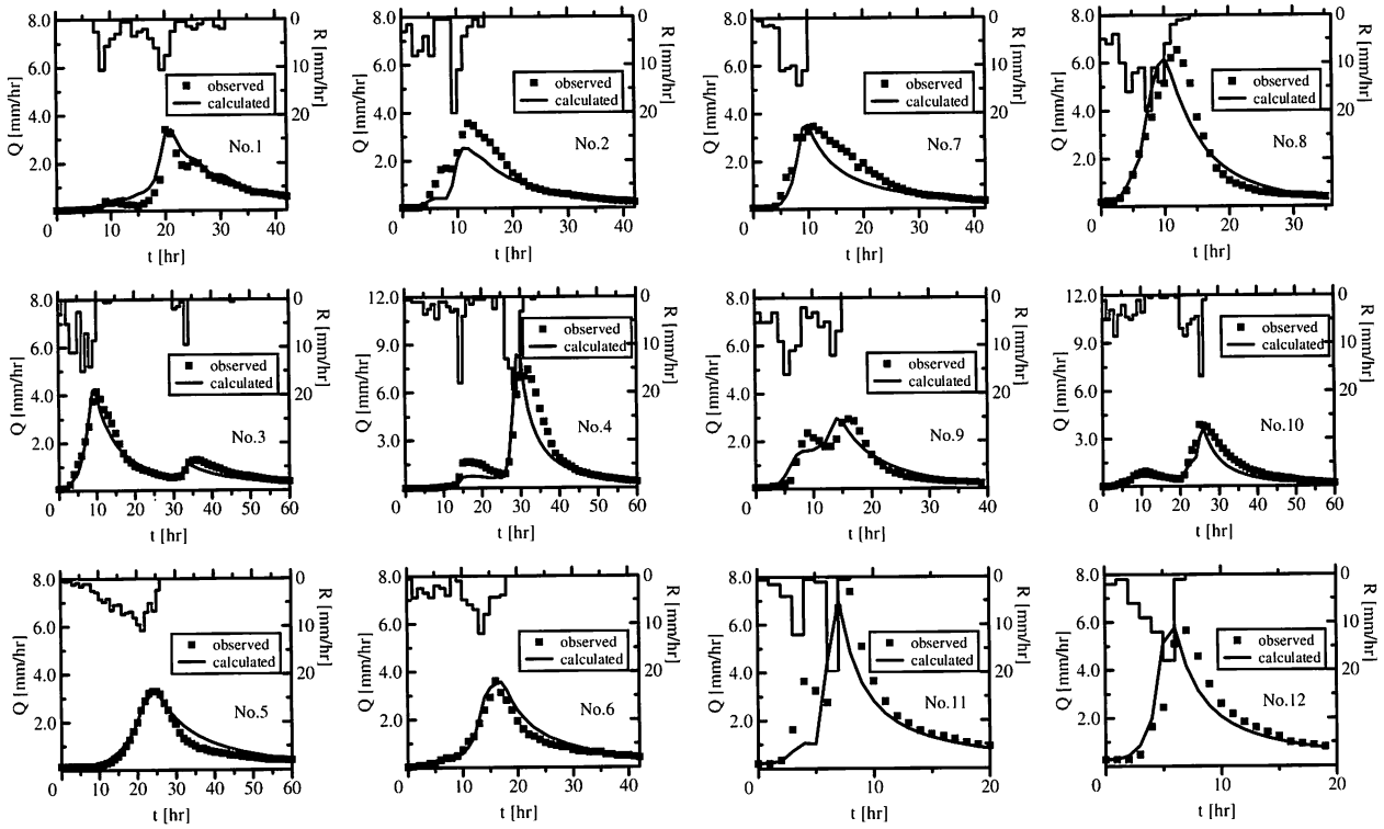
図-15 損失を考慮した貯留関数による流出量の再現計算結果の一例
