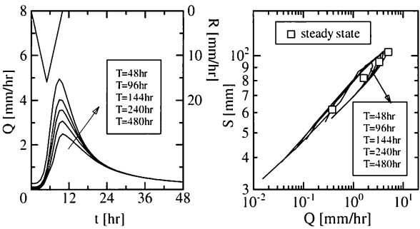
図-9 標準の流出特性値によるハイドログラフと S-Q 曲線の例 ( T は全層が湿潤した状態からの排水時間を示す)
