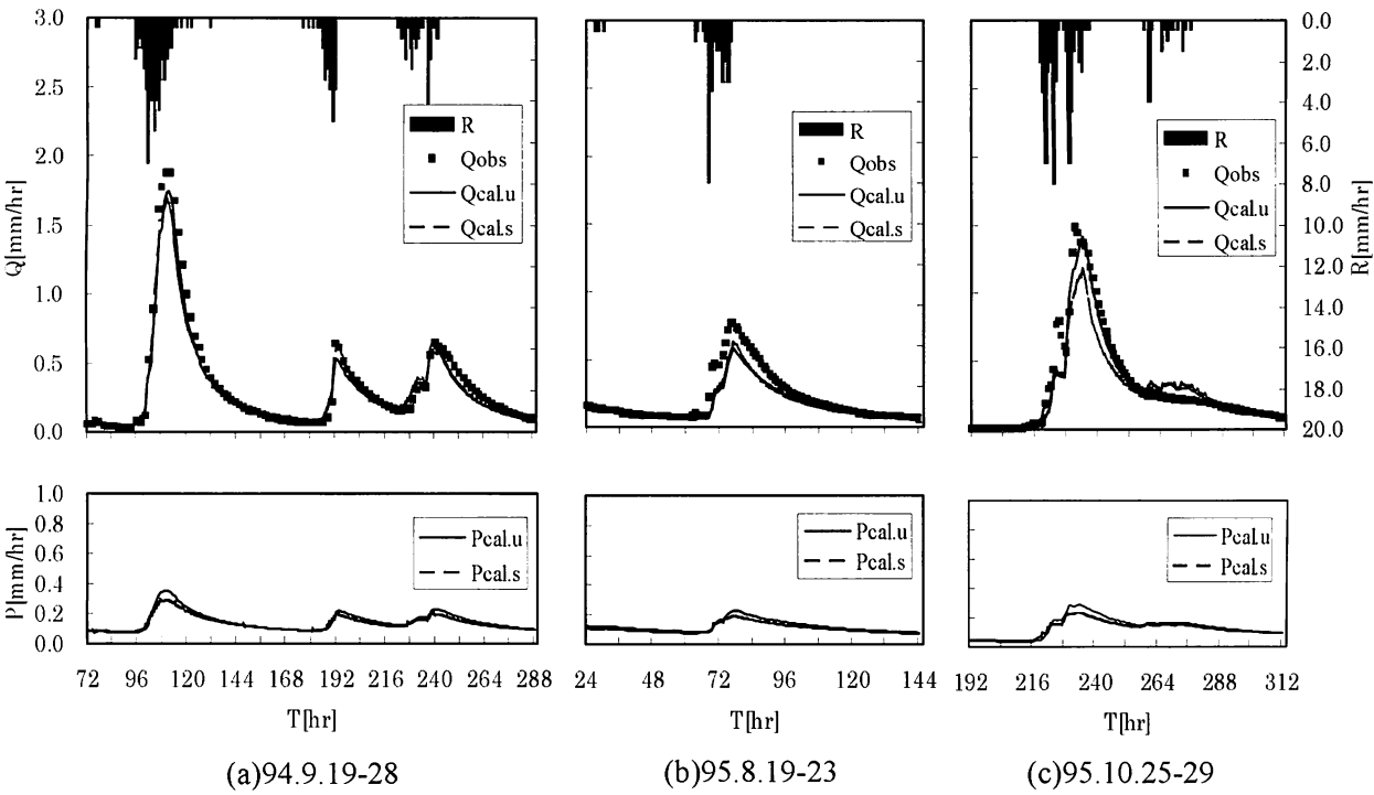
図-14 損失を考慮した貯留型流出モデルによる流出量・損失量の計算結果, 上中の沢上流域,(a)94 年 9 月 (b)95 年 8 月 (c)95 年 10 月, 上段:全流出量, 下段:損失量 (添字 u,s はそれぞれ不飽和浸透理論・貯留型モデルによる結果を示す)
