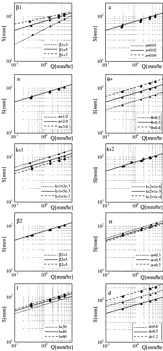
図-10 各流域条件のもとでの定常状態における S-Q 曲線の適合性
