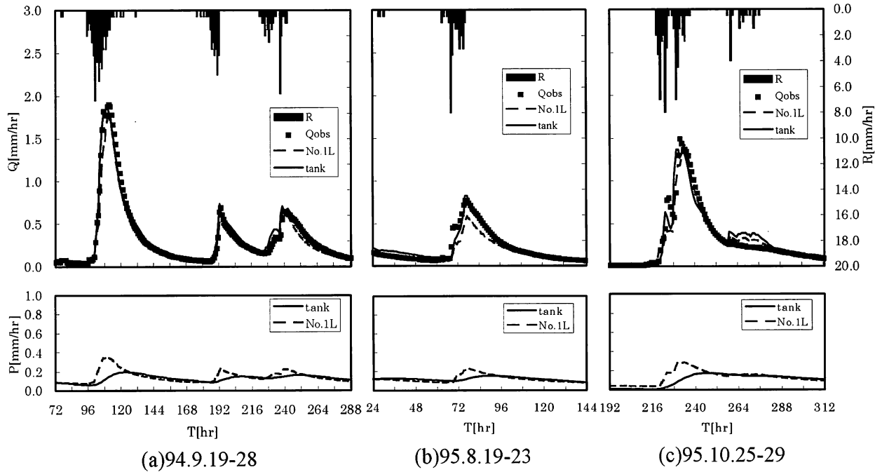
図-6 タンクモデルと不飽和浸透理論の計算結果の比較、(a)94年9 失量)
