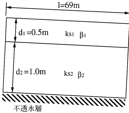
図-3 モデル化した流域の土壌構成
