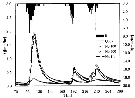
図-4 流出量の再現結果 (図中の Run-No. は表-1 による)
