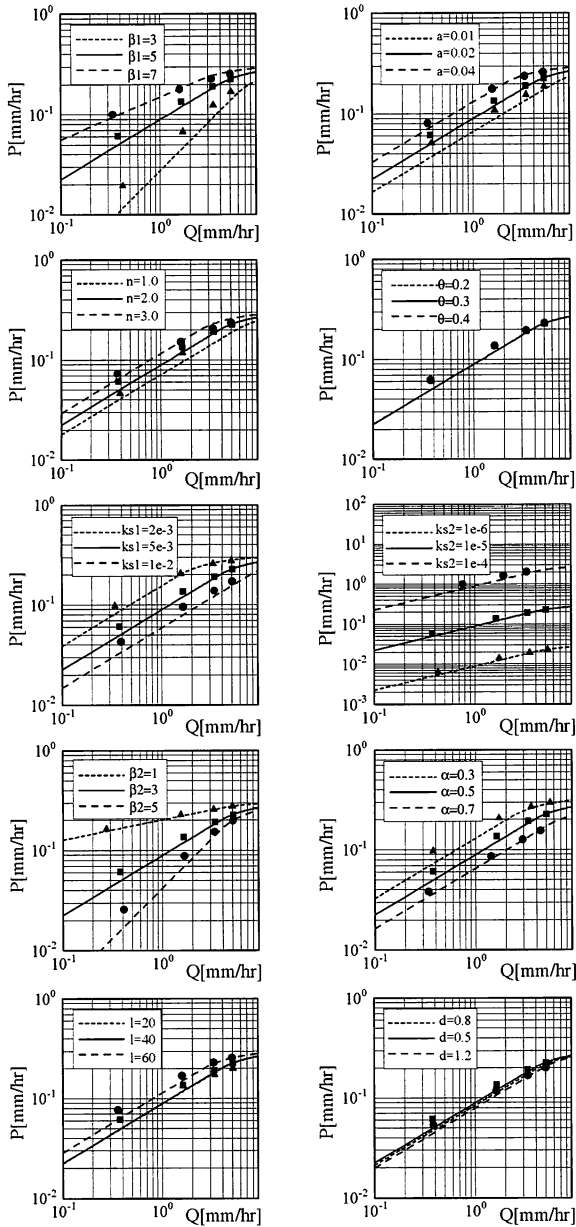
図-12 各流域条件下での定常状態における P-Q 曲線の適合性
