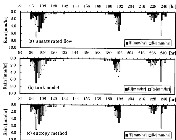
図-8 不飽和浸透理論・タンクモデル・エントロピー法による有効雨量の分離結果(上中の沢上流域, 94年9月19日～26日: (a) 不飽和浸透理論 (b) タンクモデル (c) エントロピー法)
