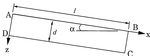
図-2 不飽和浸透理論の計算斜面
